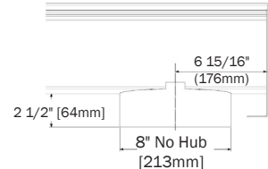
P6081N-BO8 P6083N-BO8 P6085N-BO8
