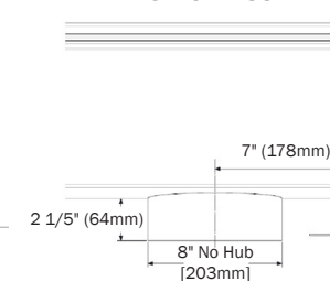
P6121N-BO8 P6123N-BO8 P6125N-BO8
