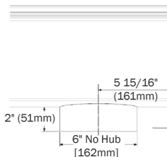
P6121N-BO6 P6123N-BO6 P6125N-BO6
